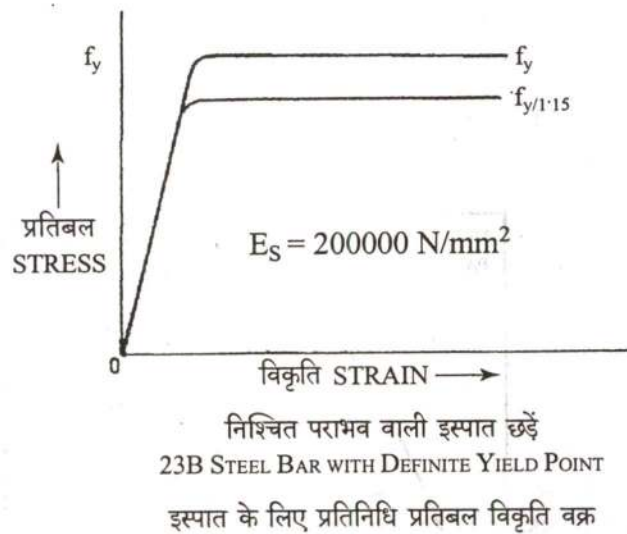
इस्पात के लिए प्रतिनिधि प्रतिबल विकृति वक्र FIG. 2 REPRESENTATIVE STRESS-STRAIN CURVES FOR REINFORCEMENT
